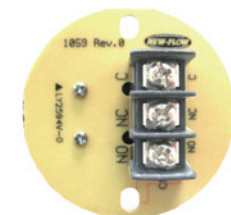
1 SPDT
